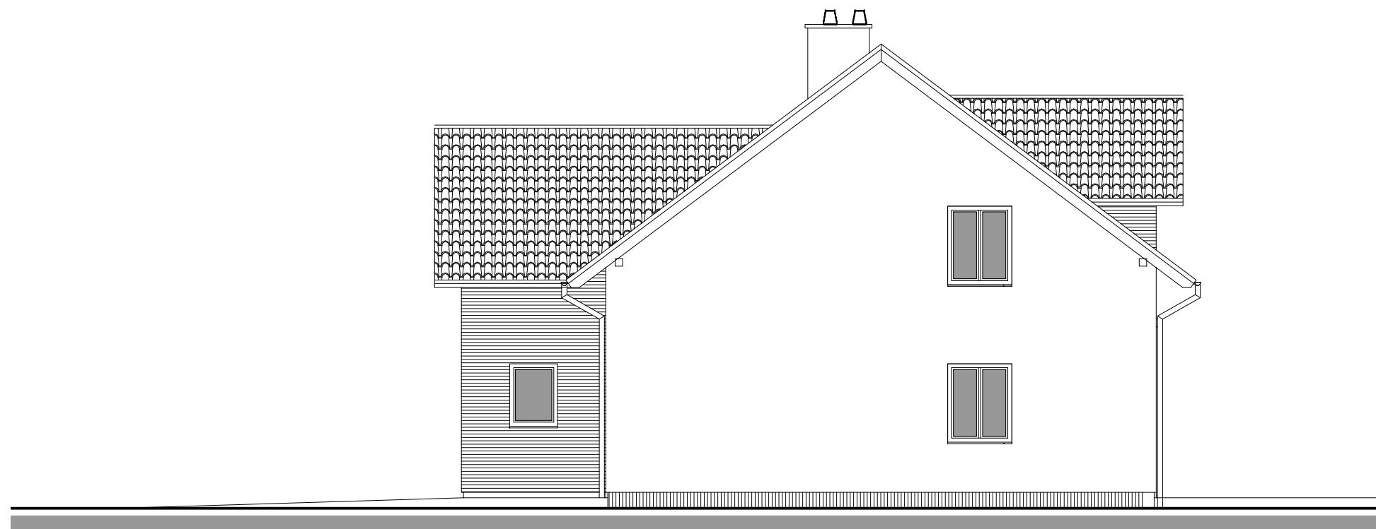
ELEWACJA PÓŁNOCNA
